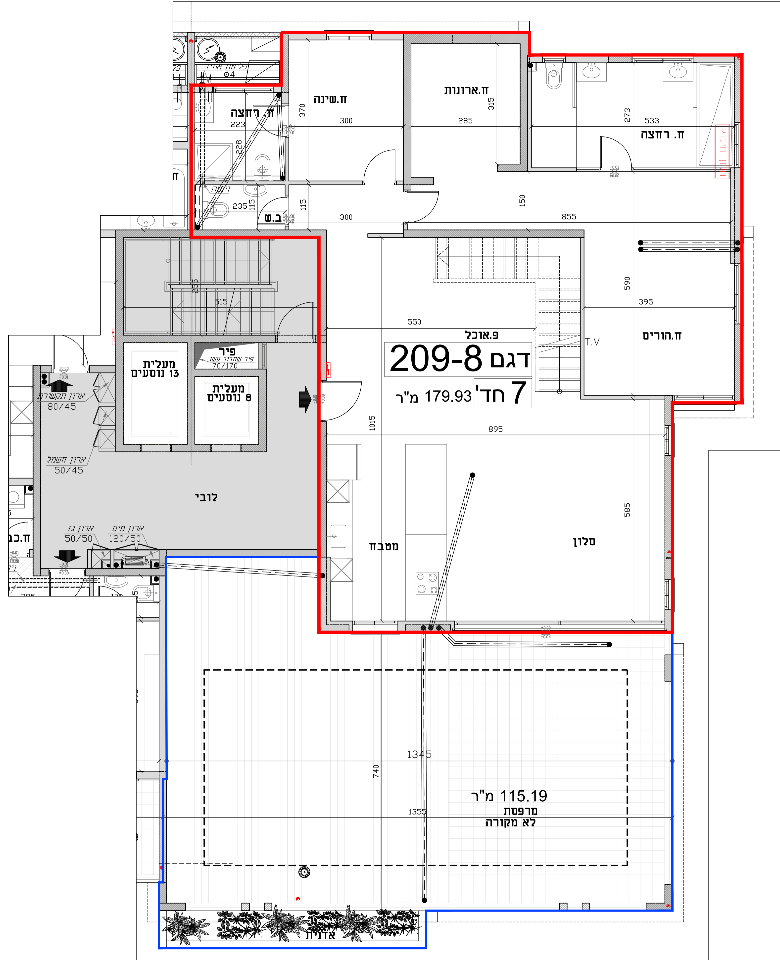
תכנית קומת פנטהאוז-8 קנ"מ 1:50
